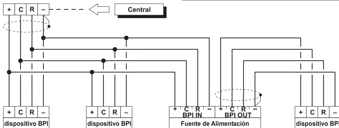
Figura 8 Conexión de 4 Dispositivos BPI.
