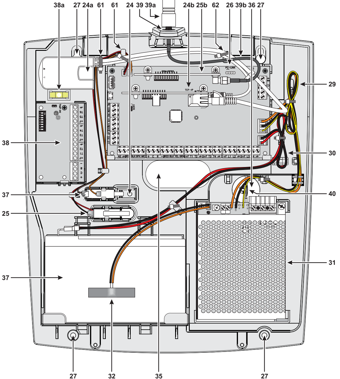
Figura 3 Partes de la central ABSOLUTA en el contenedor plástico.
