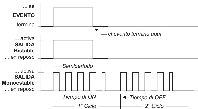
Figura 25 Efecto de los parámetros de Semiperíodo y Ciclos en las salidas Biestable y Monoestable.
