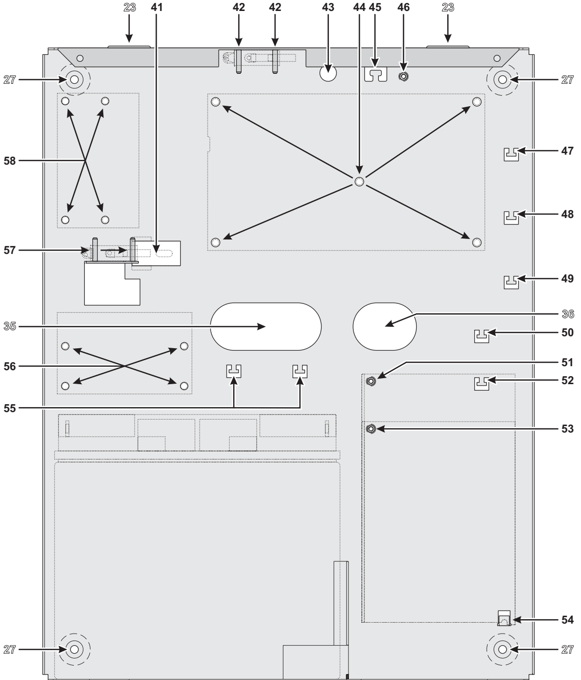
Figura 4 Fijación del contenedor Metálico.
