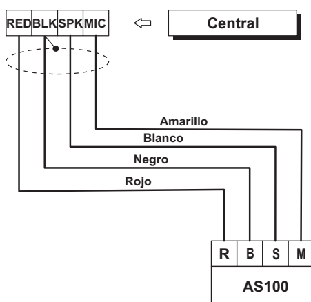
Figura 20 Conexión de l'AS100 a la central.
