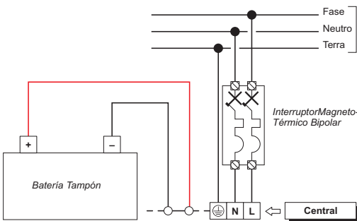
Figura 21 Conexión de la alimentación.
