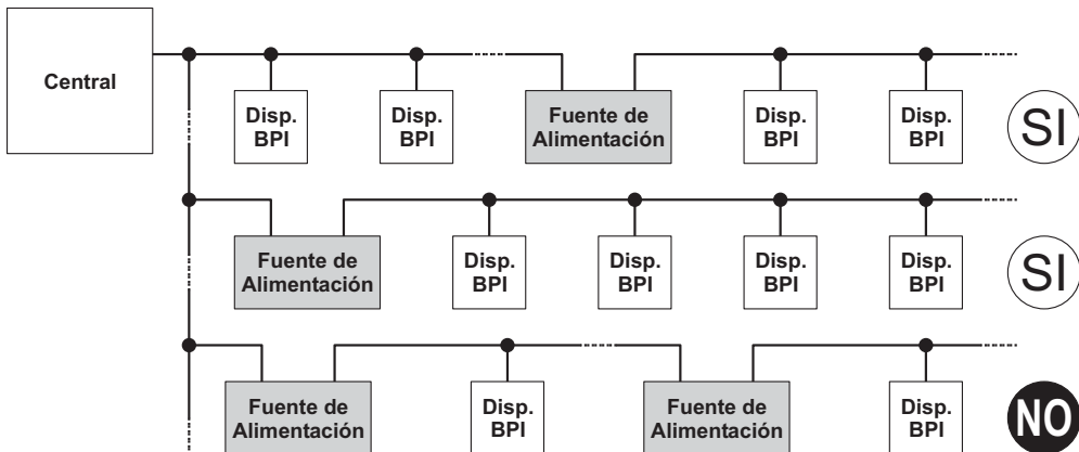
Figura 9 Conexión de las Fuentes de Alimentación
