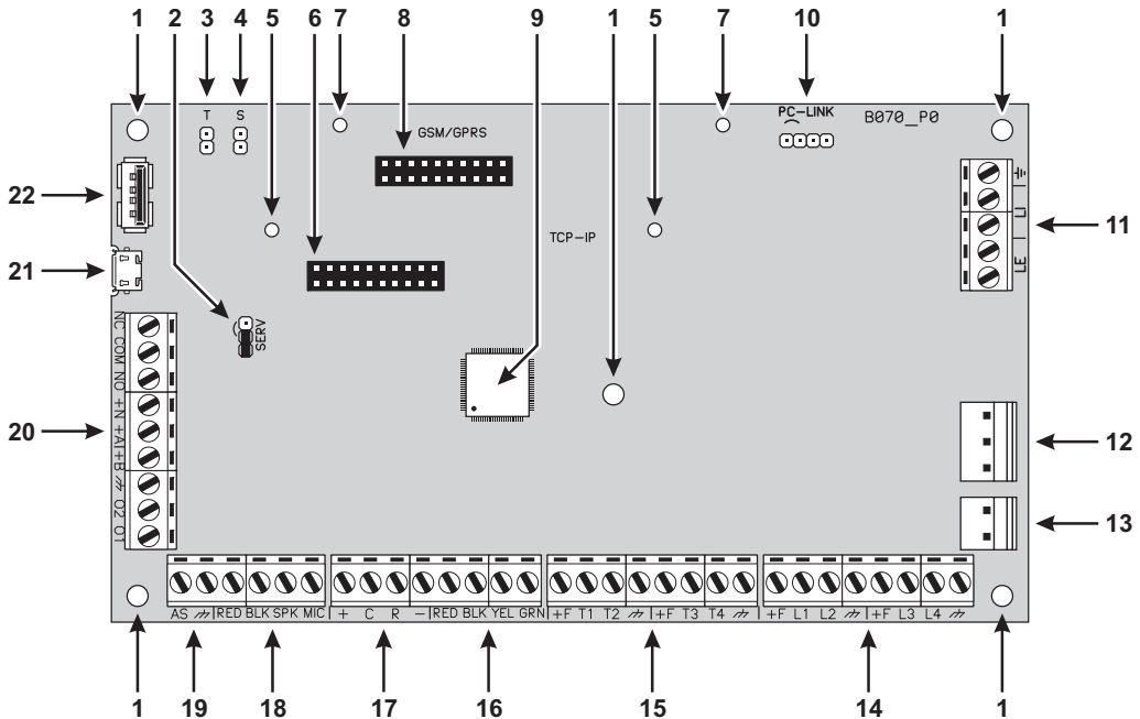
Figura 1 Placa Principal central ABSOLUTA.
