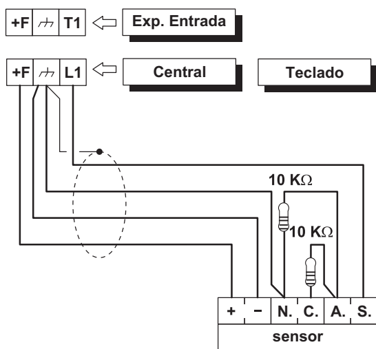
Figura 12 Conexión de un sensor a una Zona con Balance Normalmente Doble (DEOL supervisión).
