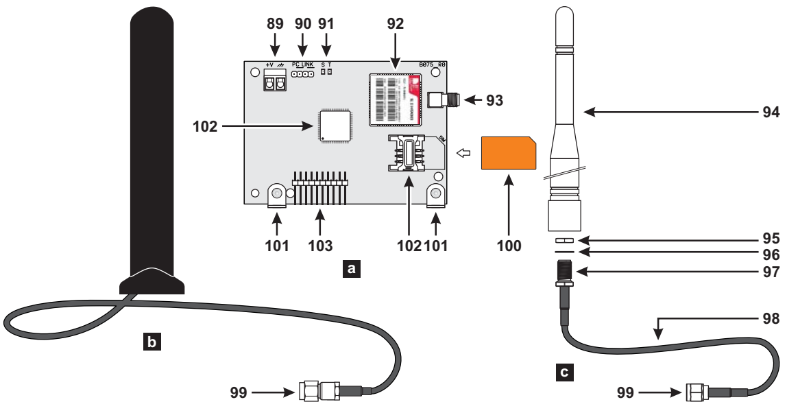
Figura 6 Partes del Módulo GSM, ABS-GSM (a), de la antena para contenedor metálico, BGSM-100CA (b), de la antena para contenedor de plástico, ABS-AK (c).
