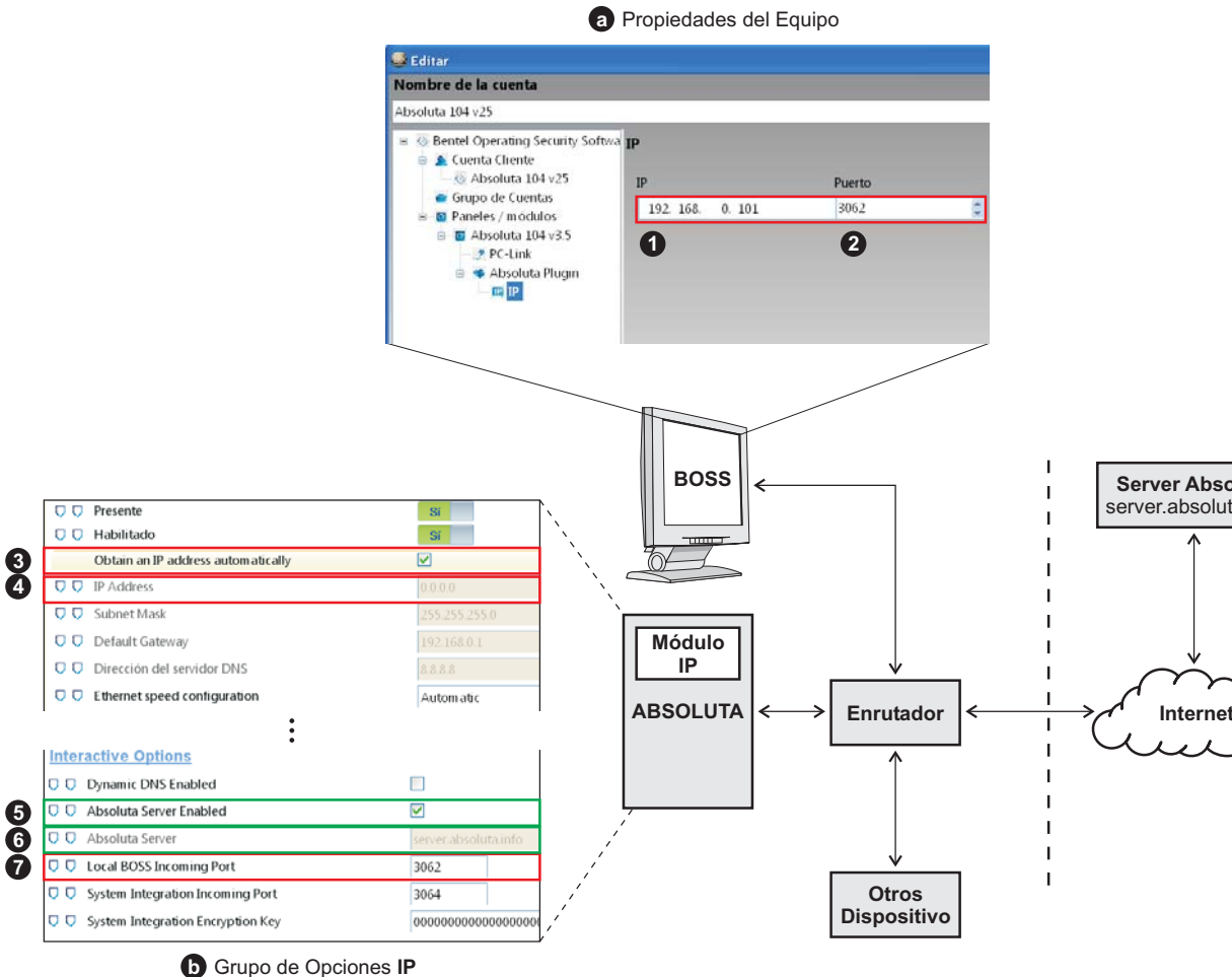
Figura 29 Conexión vía IP.
