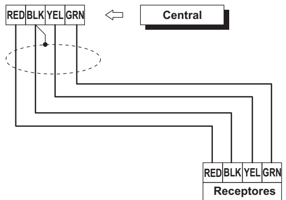
Figura 28 Conexión del Receptor a la Central.
