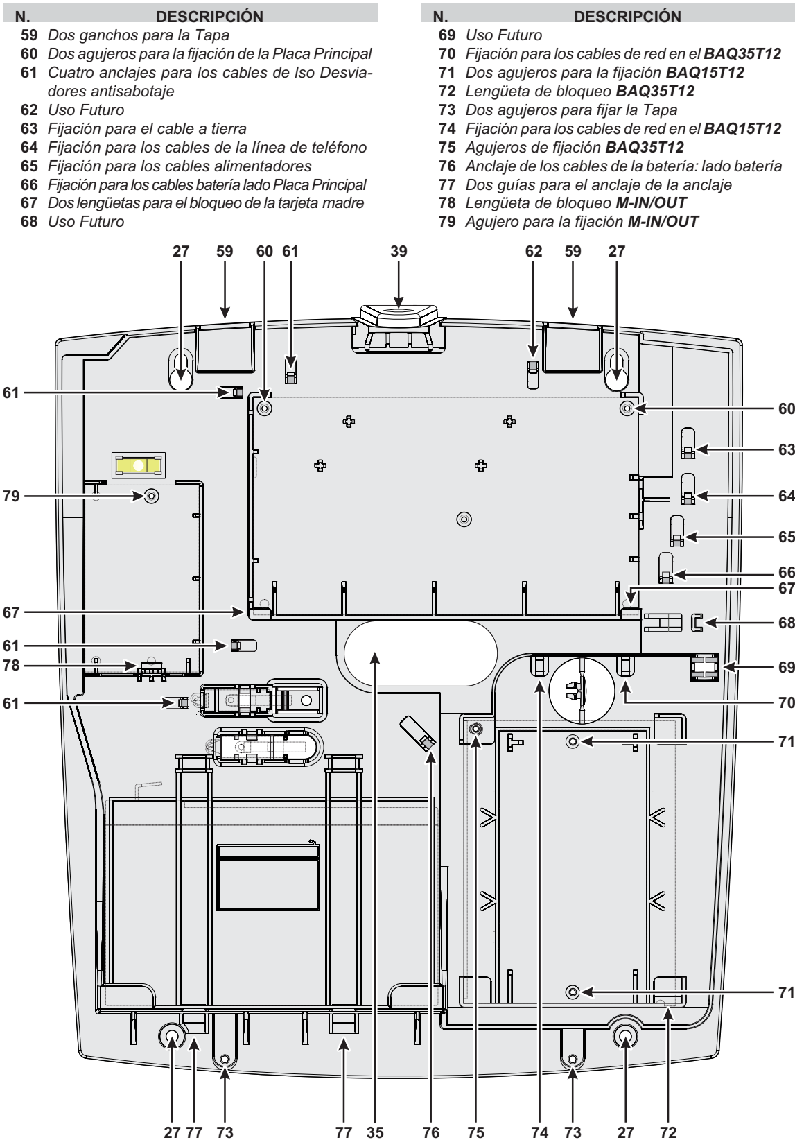
Figura 5 Fijación del contenedor Plástico.
