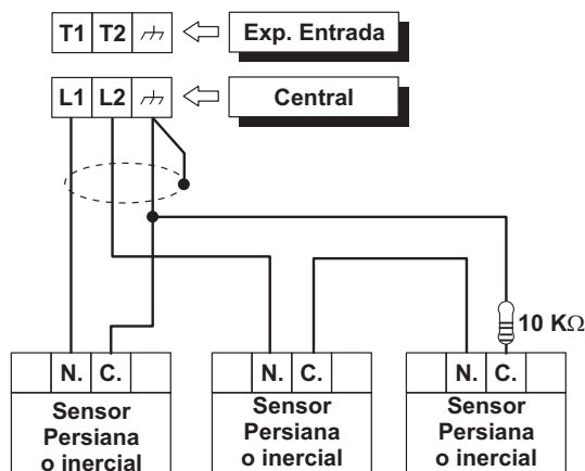
Figura 13 Conexión de sensores Inerciales (sólo para las zonas de la central) y Contactos para Persianas: conexión de un sensor a una zona N.C. de dos sensores a una zona Balanceada 10K.
