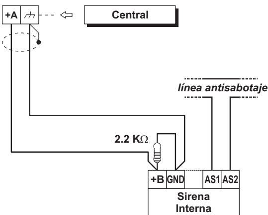
Figura 16 Conexión de una Sirena Interna a una salida Supervisada por la Centrale.
